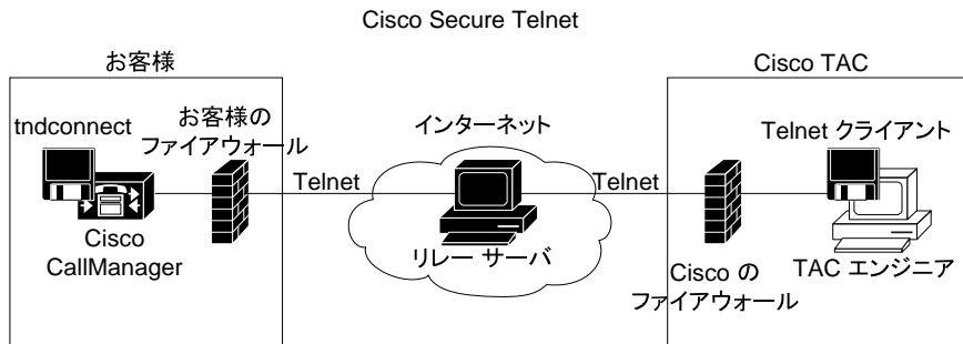
図 A-1 Cisco Secure Telnet システム
