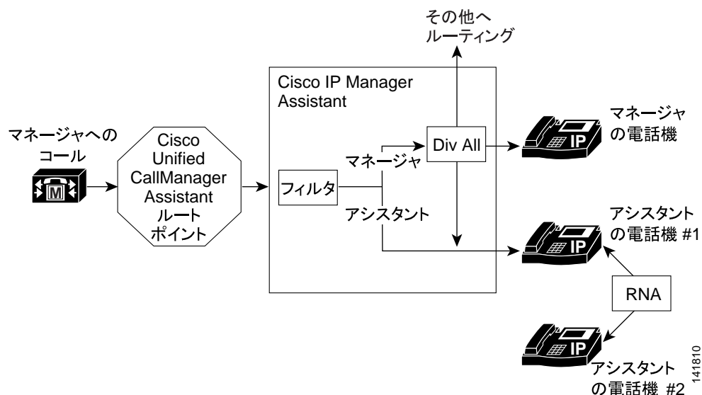
図 9-2 プロキシ回線サポート用の Cisco Unified Communications Manager Assistant のルーティングロジック
