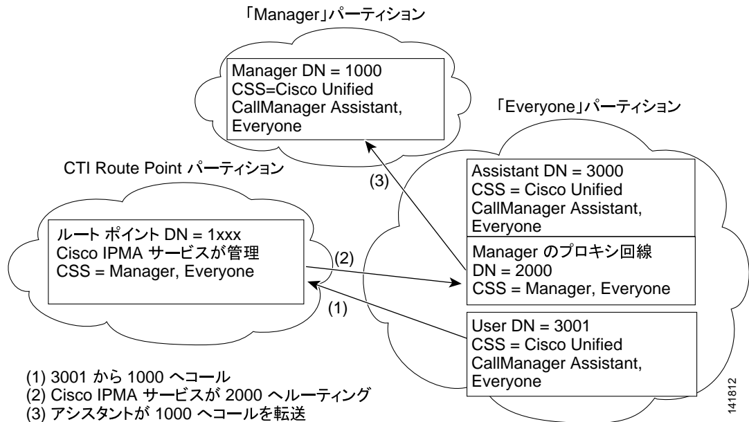
図 3-4 プロキシ回線サポート用の Cisco Unified CallManager Assistant のコーリング サーチ スペースおよびパーティションの設定例
