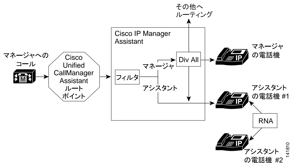
図 3-2 プロキシ回線サポート用の Cisco Unified CallManager Assistant のルーティング ロジック
