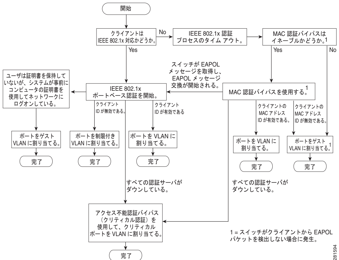
図 12-2 認証フローチャート
