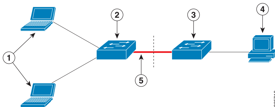
図 12-6 CISP を使用したオーセンティケータまたはサブリカント スイッチ
