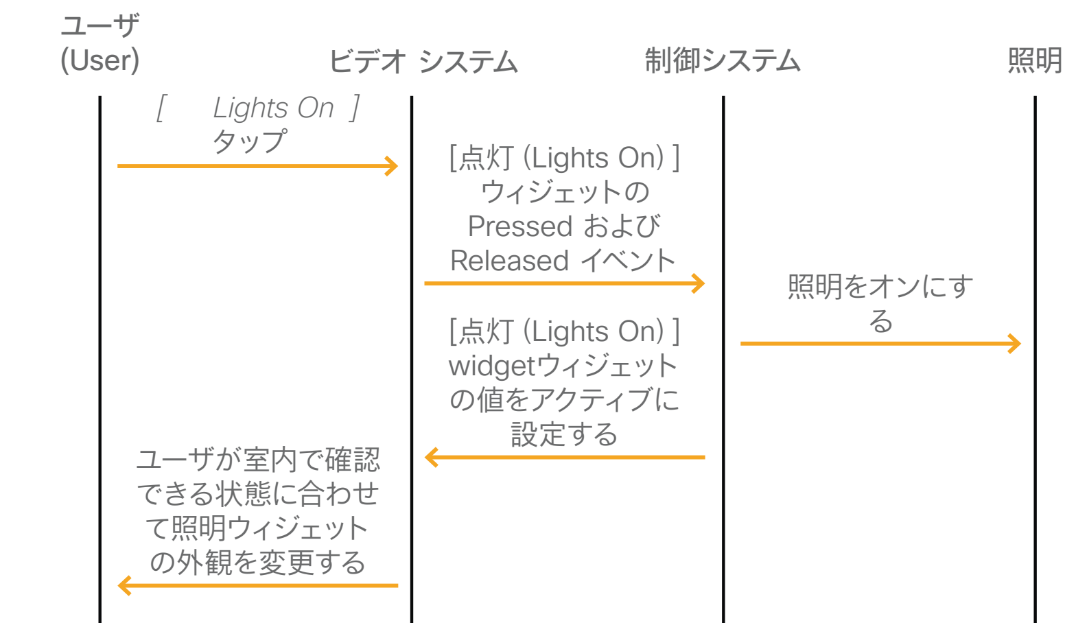
メッセージ フロー: Touch10/DX/Webex Board のコントロールを使用して照明をオンにする
