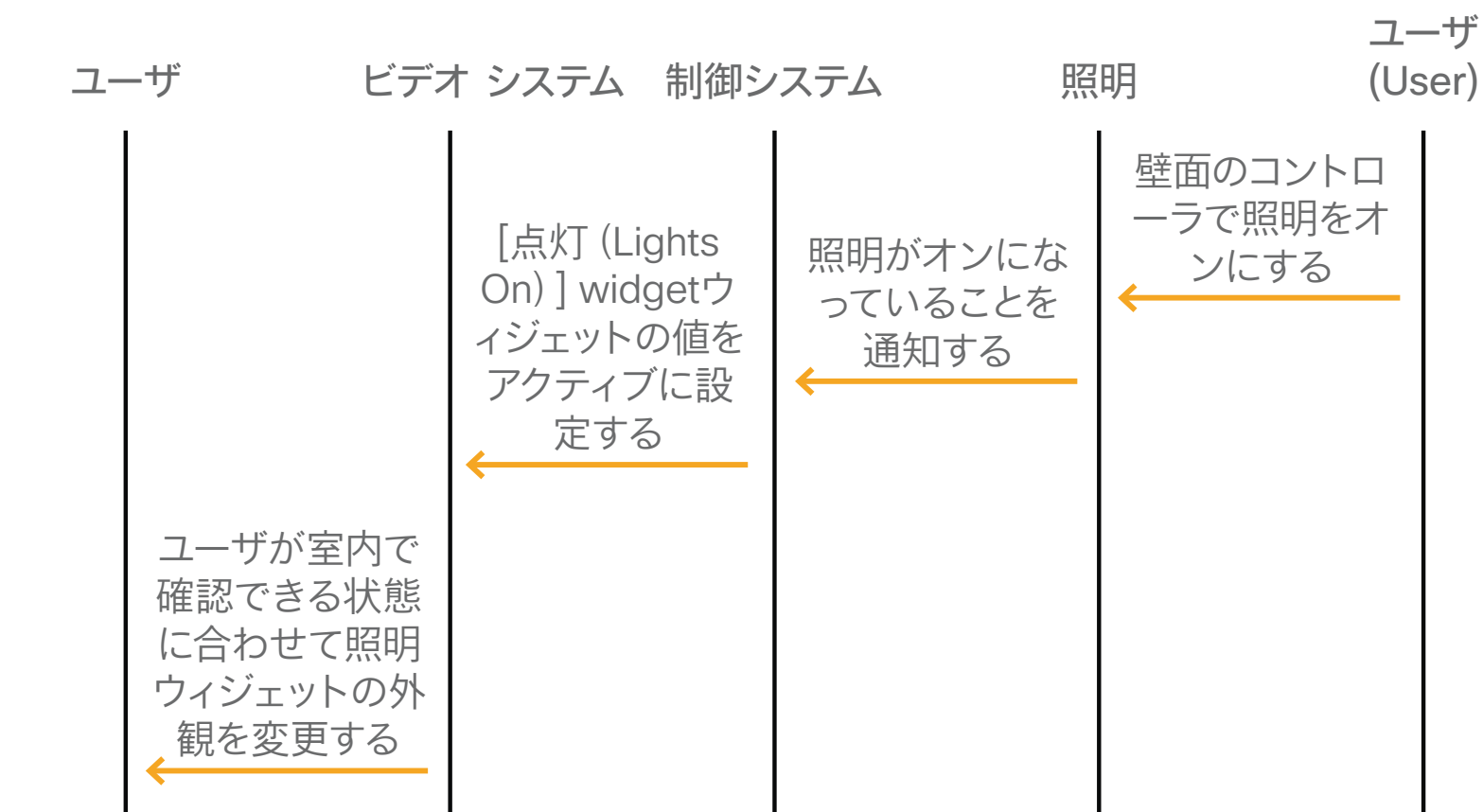
メッセージ フロー: 壁面のコントローラを使用して照明をオンにする
