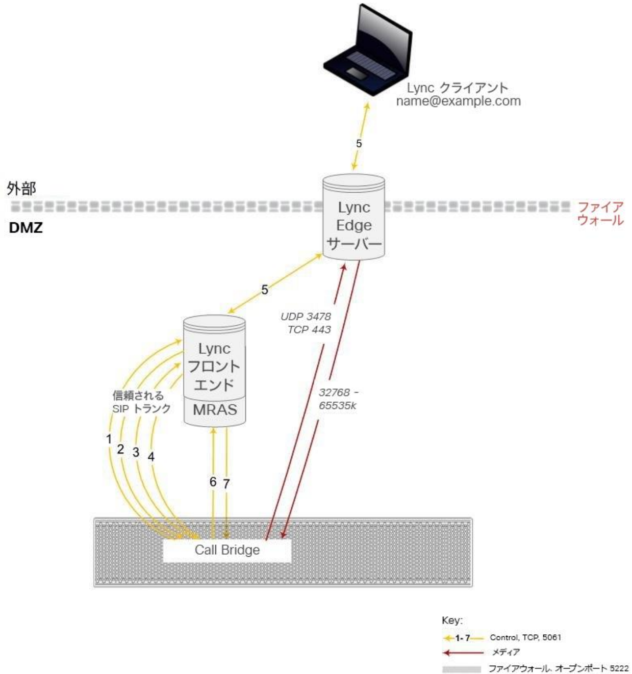
図 16 : Lync Edge サーバへの Call Bridge のコールフロー
