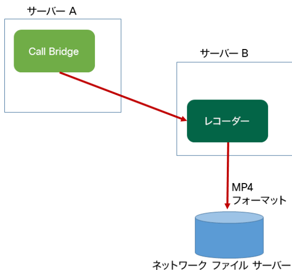
図 19：テストのみを目的として許可されている展開：ローカルモード
