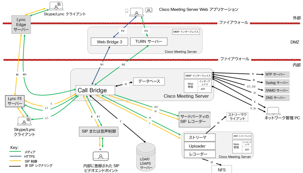
図 24 : DMZ 内の TURN サーバと Web Bridge 3 コンポーネントを使用して分散型サーバ展開で開く必要があるポート
