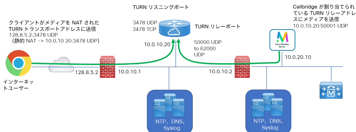
図 9 : UDP を使用した TURN のサンプル図
