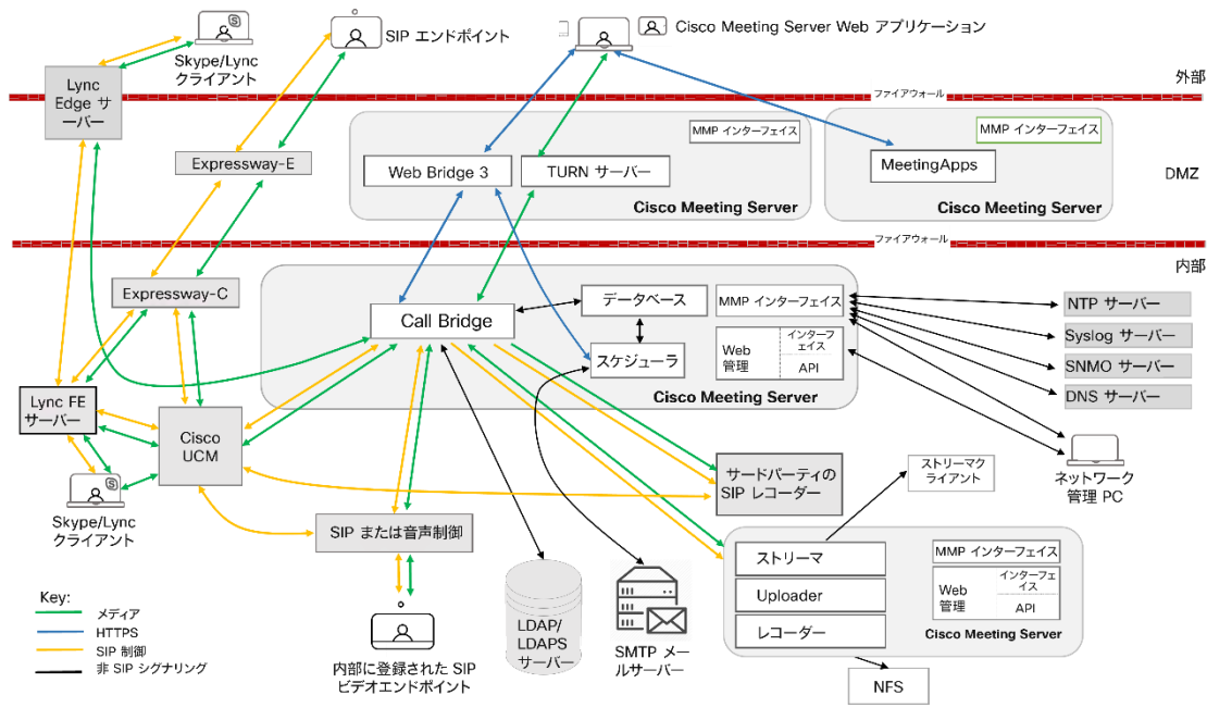
図 7：分割型サーバ展開で TURN サーバコンポーネントを使用する Meeting Server 展開例
