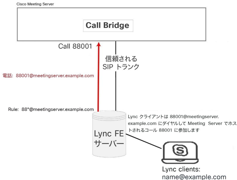
図 13 : Meeting Server でホストされたミーティングに発信する Lync クライアントの例
