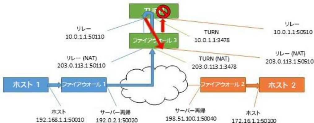
図 32 : リレー間のパスを使用したホスト間のメディアパス (NAT あり)
