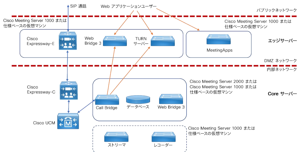
図 2 : Meeting Server Edge を使用した分割型サーバー展開
