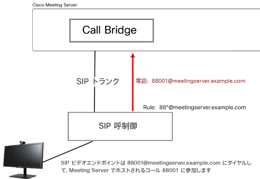
図 12 : Meeting Server でホストされたコールを呼び出す SIP ビデオエンドポイントの例
