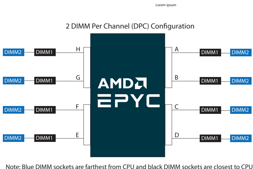
図4 8チャンネルメモリ構成
