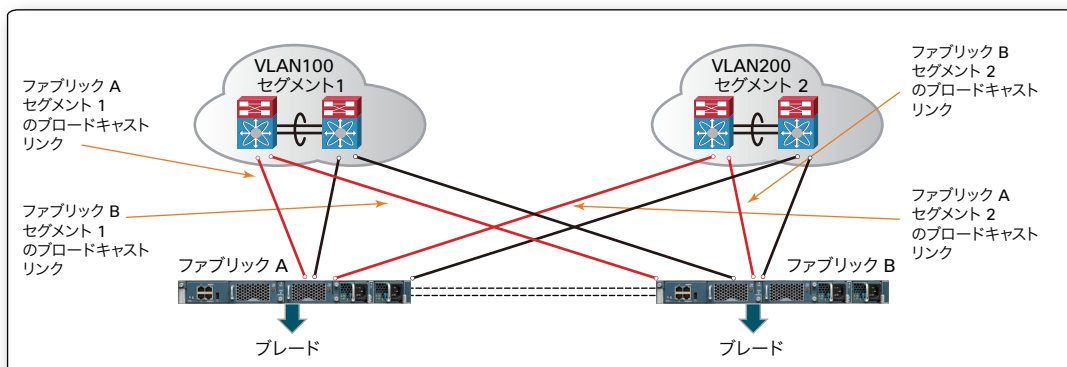
UCS 2.0 リリースのエンド ホスト モードと上位ネットワークとの接続
